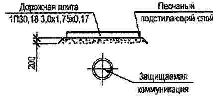
Схема защиты коммуникаций попадающих в опасную зону
