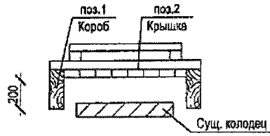
Схема защиты колодца
