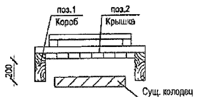
Схема защиты колодца
