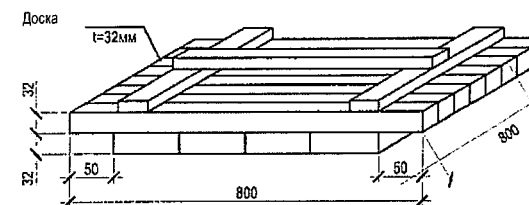
Крышка (поз.2)
