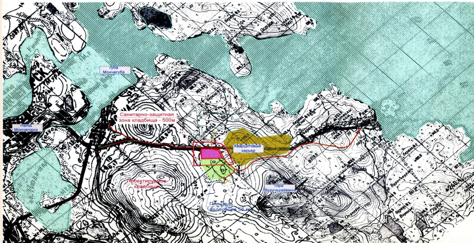
Ситуационный план М 1:50000
